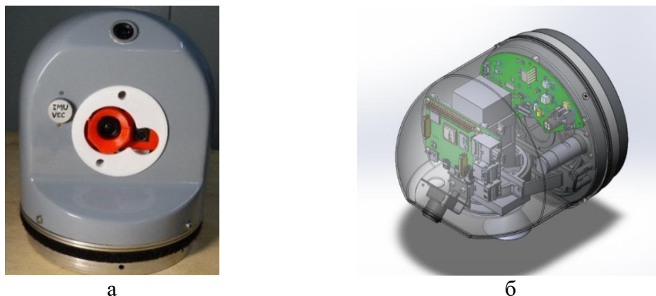
Рисунок 1 – Малогабаритная гиперспектральная камера(а) и ее твердотельная модель (б) в составе ЦН для БАК
